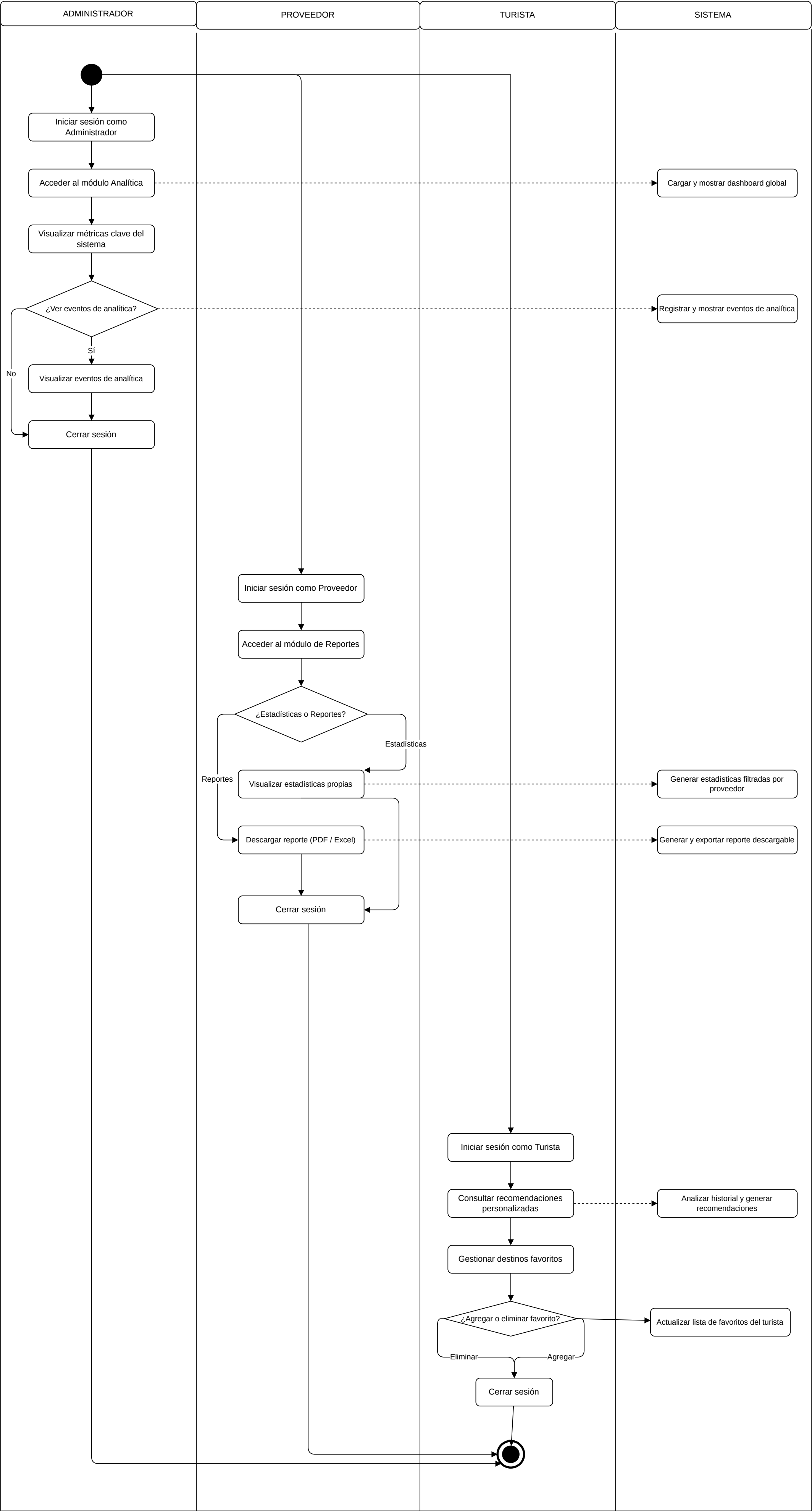
Diagrama de Actividades - RF08: Analítica, Reportes y Gestión del Negocio
